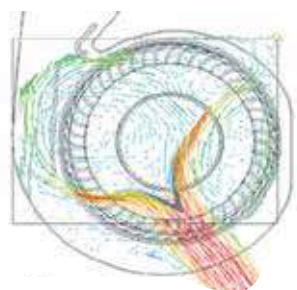
Konštrukcia s rovnomerným rozdelením vzduchu
